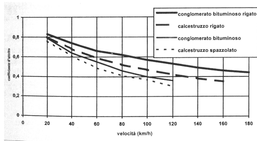
figura 4.6 Variazione del coefficiente d'attrito su piste di volo bagnate di diverso tipo al variare della velocità.
