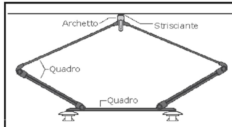
Disegno semplificato del pantografo
