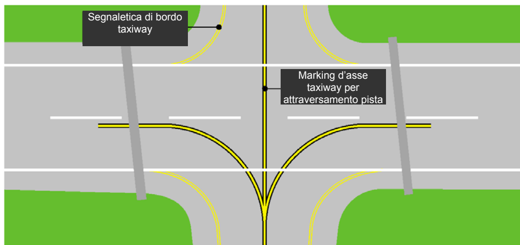
Figura 7.20 – Markings per taxiway di attraversamento della pista
