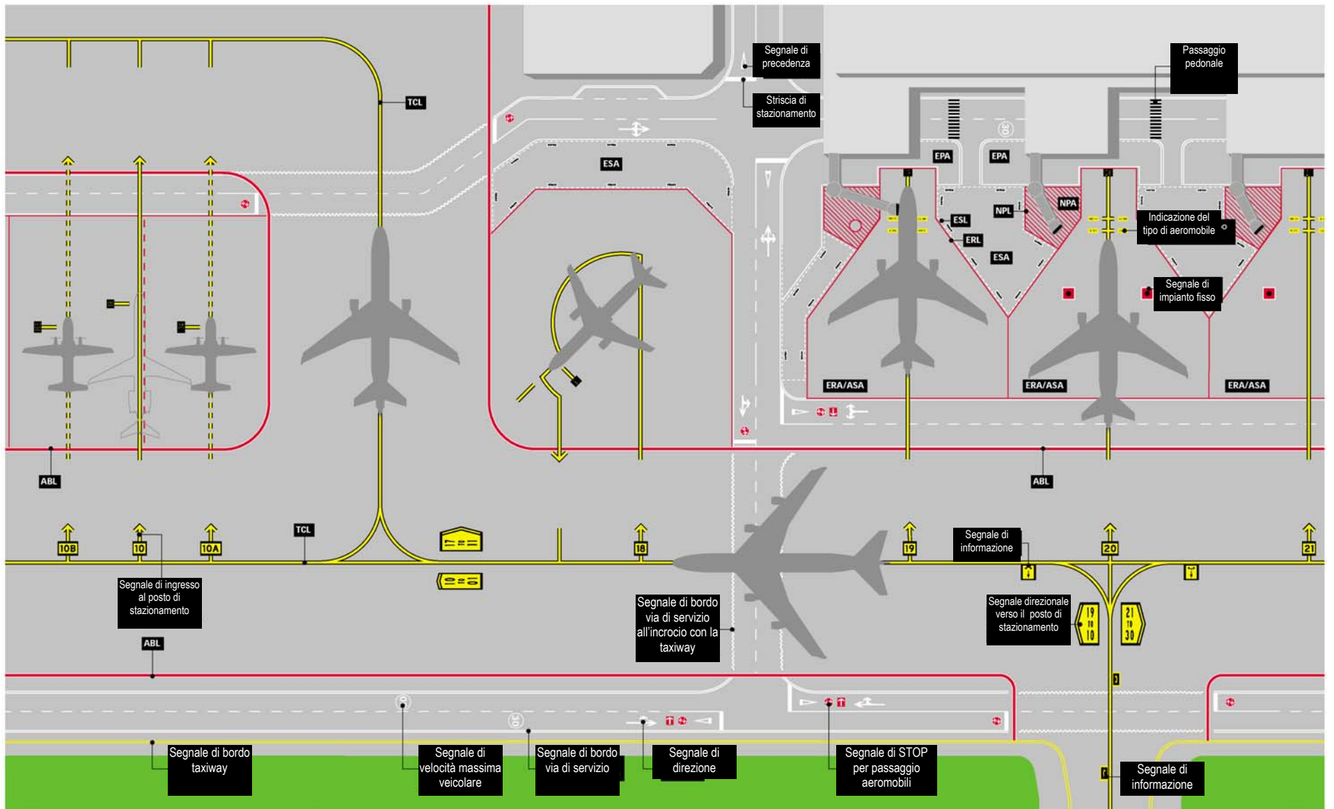
Figura 7.33 – Esempio di segnaletica di piazzale
