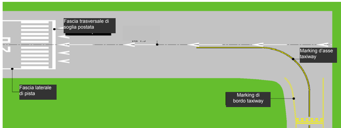
Figura 7.19 – Markings per innesto taxiway su pista con soglia spostata
