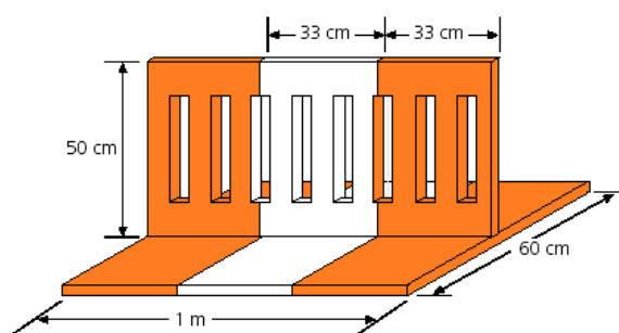
Figura 7.34 - Segnalatore di Tipo 'A' per terreno inagibile
